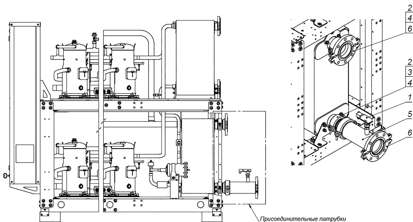
Рисунок 5.2.2. Схема сборки присоединительных патрубков гидравлического контура чиллеров.
