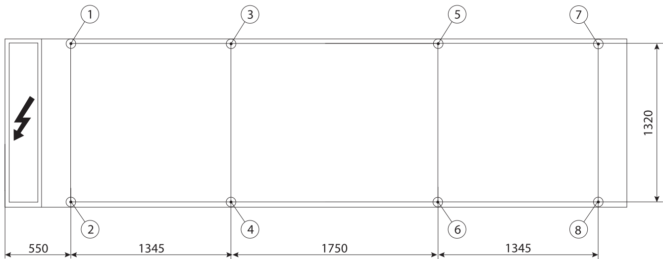
Рисунок 4.3.12. Монтаж опор и распределение нагрузки чиллера 1100
