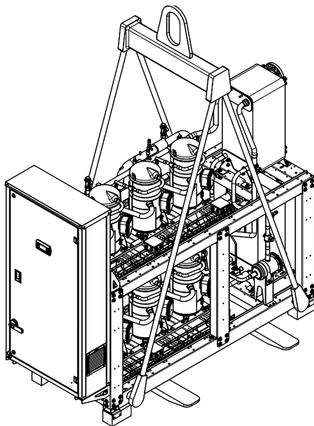
Рисунок 4.2.1. Схема строповки чиллера 320 б) изометрия чиллера 320
