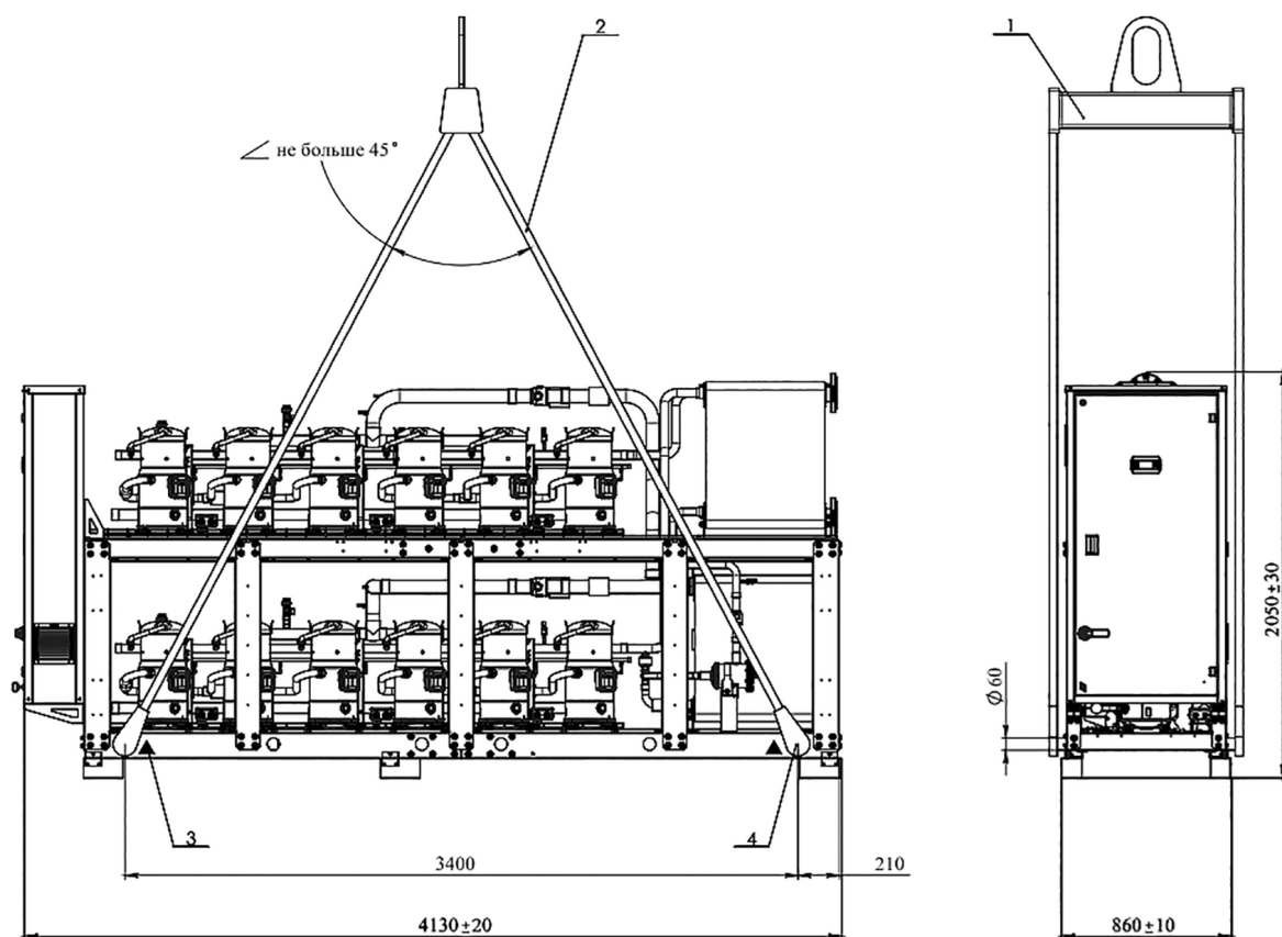
Рисунок 4.2.4. Схема строповки чиллеров 600/660
