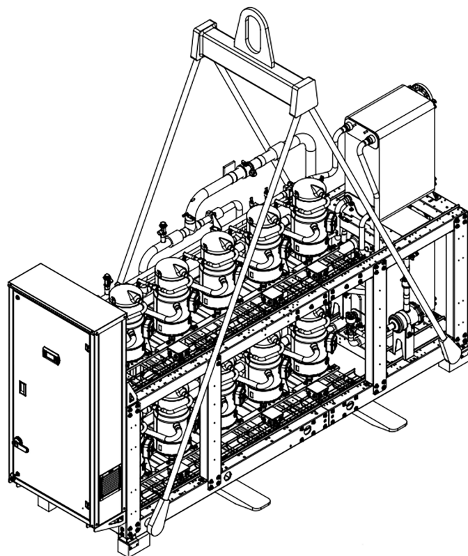
Рисунок 4.2.3. Схема строповки чиллеров 510/560
