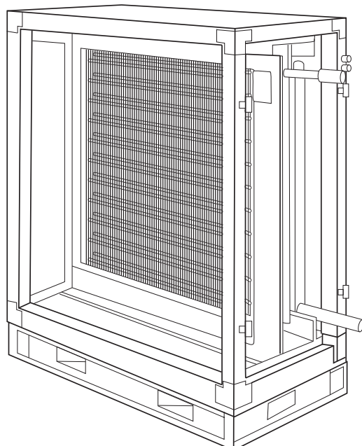
Рисунок 4. Секция воздушонагревателя водяного
