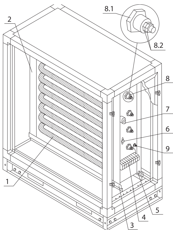
Рисунок 24. Секция воздушонагревателя электрического:
