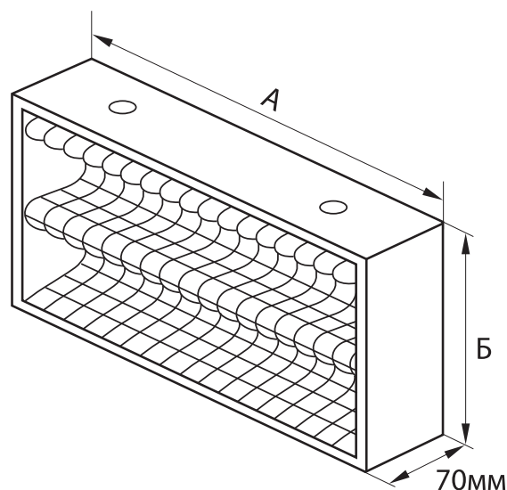
Рисунок 8. Фильтрующая вставка
