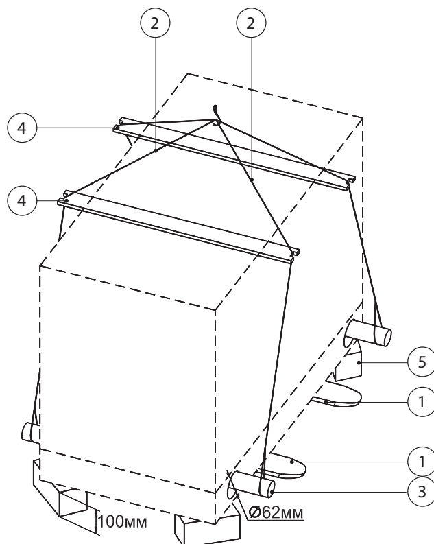
Рисунок 4.1. Схема погрузки
