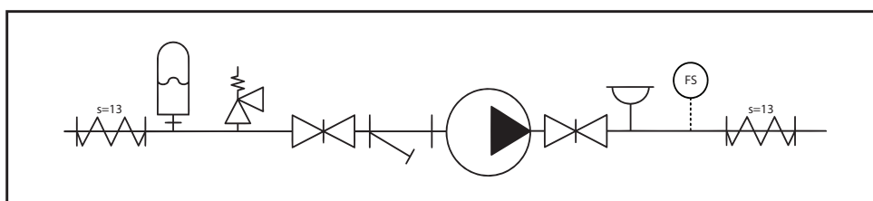
Рисунок 6.1. Схема принципиальная гидравлического контура гидромодуля с одним насосом
