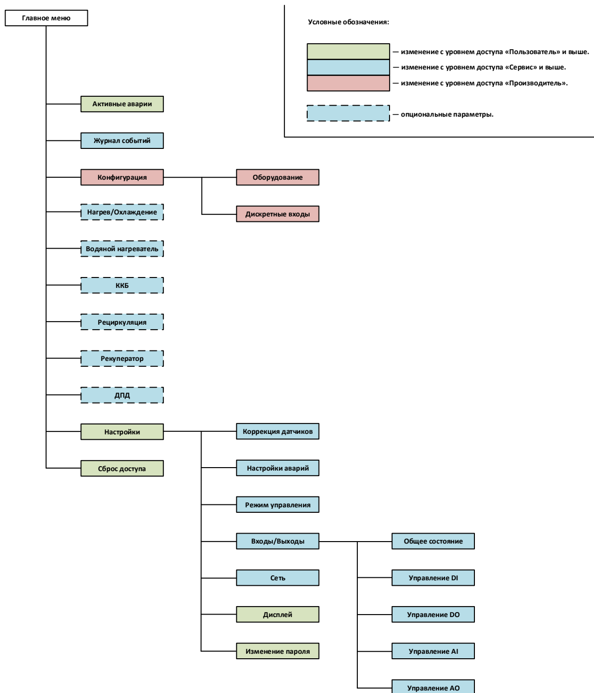
Рис.4. – Структура меню Zentec.
