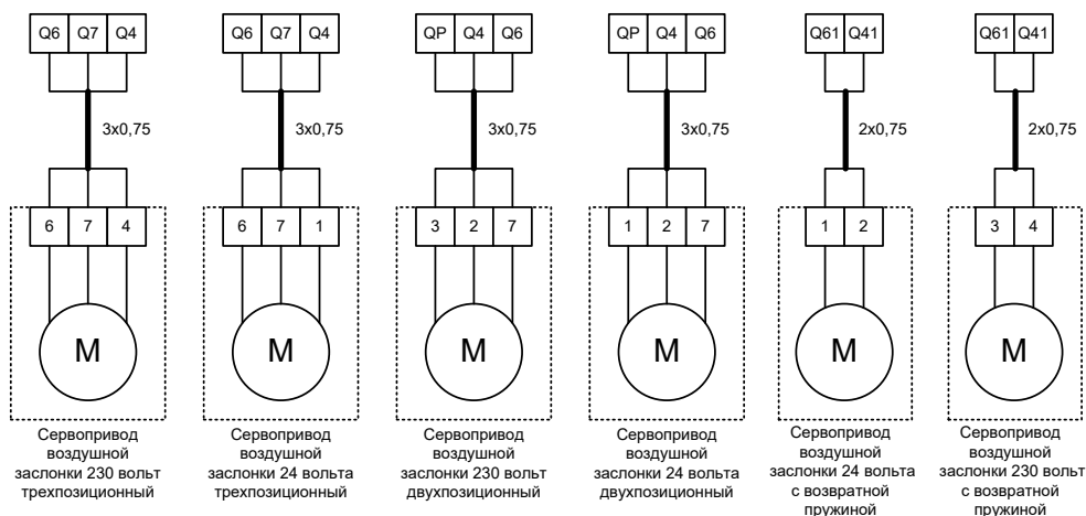
Рисунок 25. - Подключение заслонок наружного воздуха.
