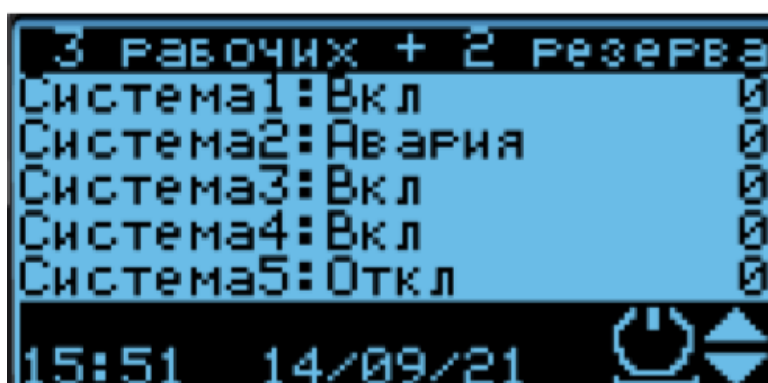
Рис.5.- Главное меню контроллера.
