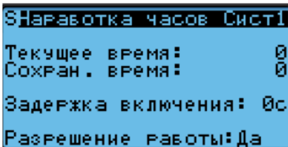
Рис.14.- Настройка времени задержки включения
