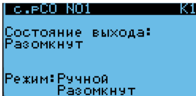
Рис.10.- Выходы реле
