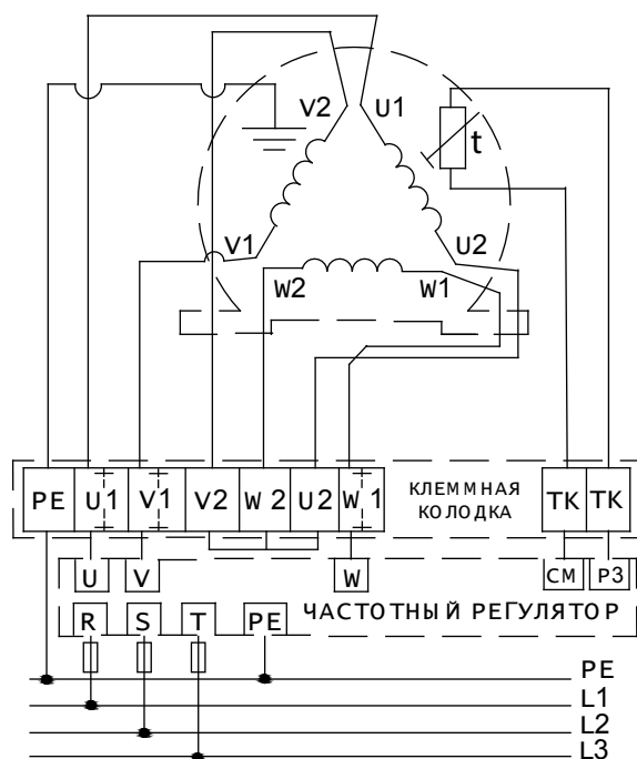
Рисунок 8. Схемы подключения электродвигателей вентиляторов
