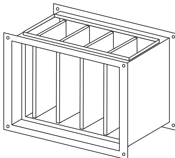
Рисунок 60. Карманный фильтр
