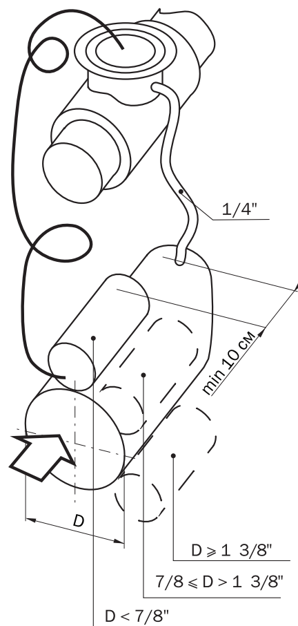
Рисунок 42. Крепление термобаллона
