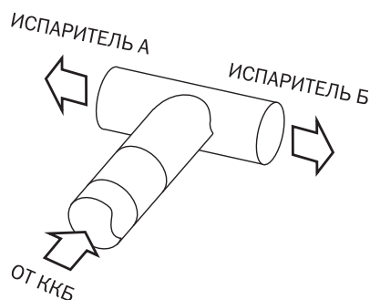
Рисунок 43. Тройник (рефнет-разветвитель)
