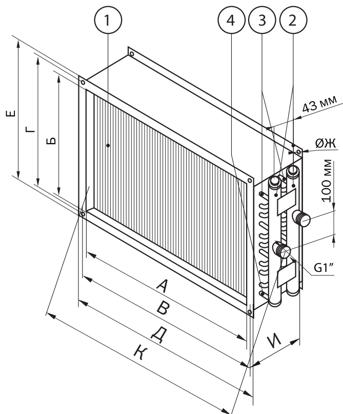
Рисунок 17. Устройство водяных воздушонагревателей:
