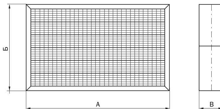
Рисунок 59. Внешний вид кассетных вставок
