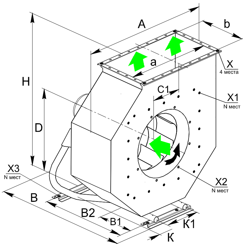
Рисунок 1. Общий вид вентилятора стандартного исполнения (направление вращения рабочего колеса – левое (L))
